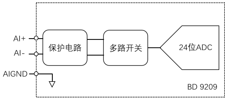
BD 9209 某通道的电路示意图
